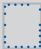
Systemdarstellung RC3 19 Verriegelungspunkte hochwertiger RC3 Beschlag systemgerechte Schrauben Schließbleche aus gehärteten Stahlloberteilen (auch erhältlich als WinTech Secure 3*)
